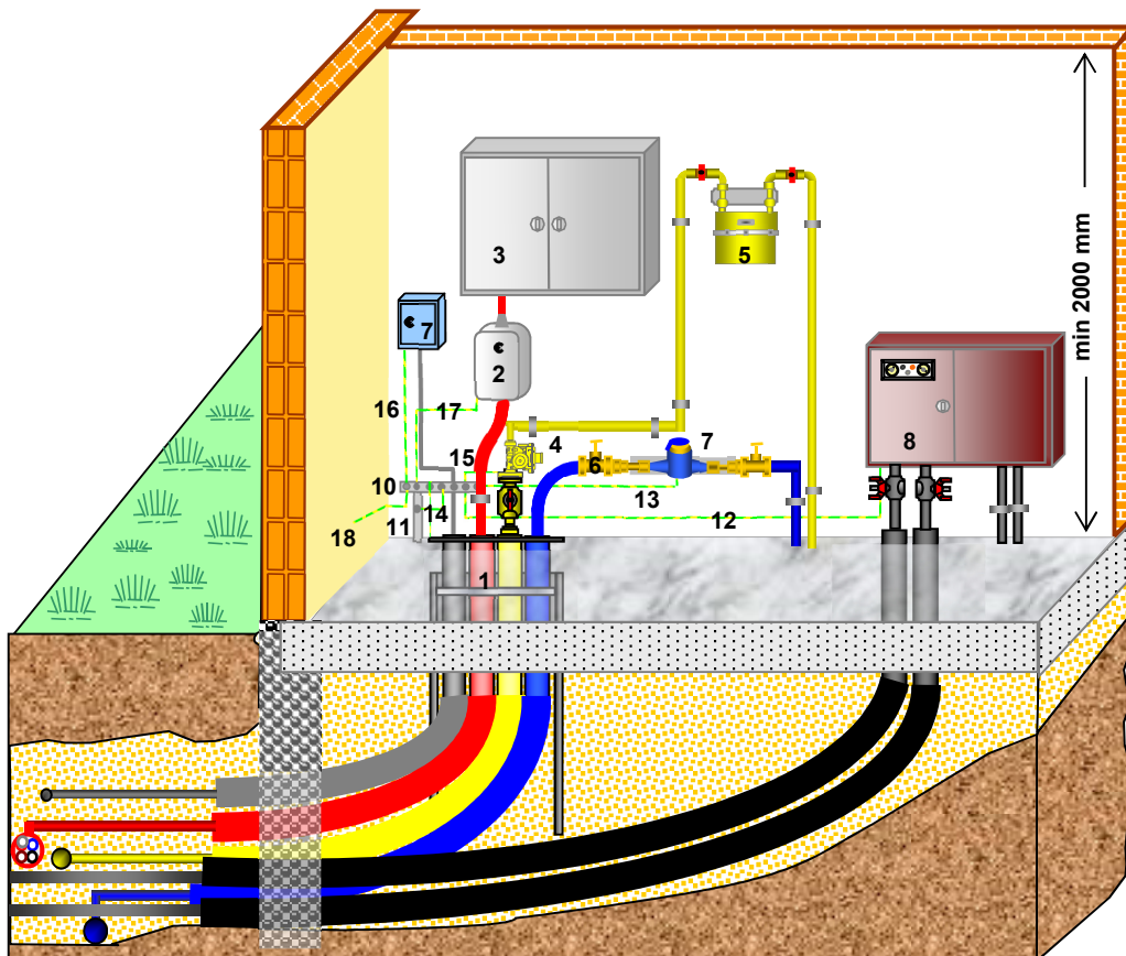
Abbildung 2: Die Hausanschlusswand für Gebäude mit ≤ 4 Wohneinheiten (Beispiel eines nicht unterkellerten Gebäudes)
